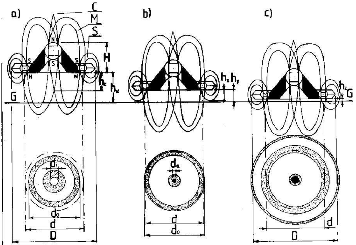
Rys. F33. Zależność kształtu lądowiska pojedynczego magnokraftu od głębokości lądowania.
